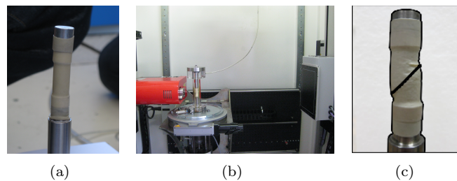
FIGURE 1 – (a) Un échantillon cylindrique de sable avant le test de compression triaxiale, (b) une expérience du test de compression avec acquisition d'une séquence d'images 3D, et (c) la bande de cisaillement observée après le test de compression.
