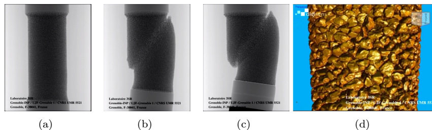
FIGURE 2 – (a, b, c) Scans 3D à plusieurs reprises au cours du test de compression, et (d) la visualisation 3D
