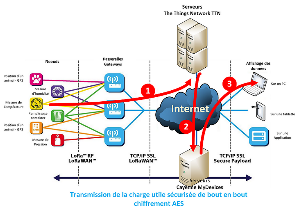
Figure 2 : Architecture LoRa de bout en bout
