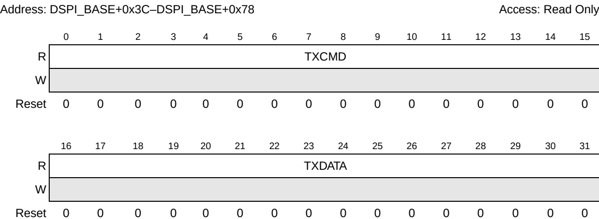
Figure 25-10. DSPI Transmit FIFO Register 0–15 (DSPI_TXFR0–DSPI_TXFR15)
