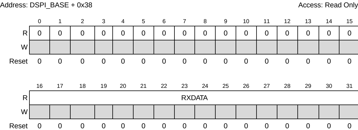
Figure 25-9. DSPI POP RX FIFO Register (DSPI_POPR)
