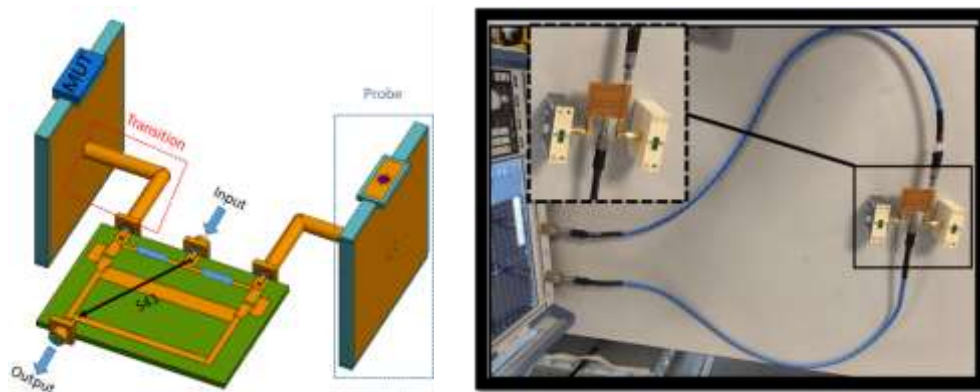
Figure 2 : Structure différentielle pour la détection du cancer de la peau. A gauche, principe de fonctionnement et accès de mesure, à droite banc de mesure.
