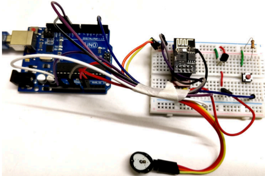
Figure 2. Système de surveillance des patients basé sur l'IOT utilisant l'ESP8266 et l'Arduino [2].
