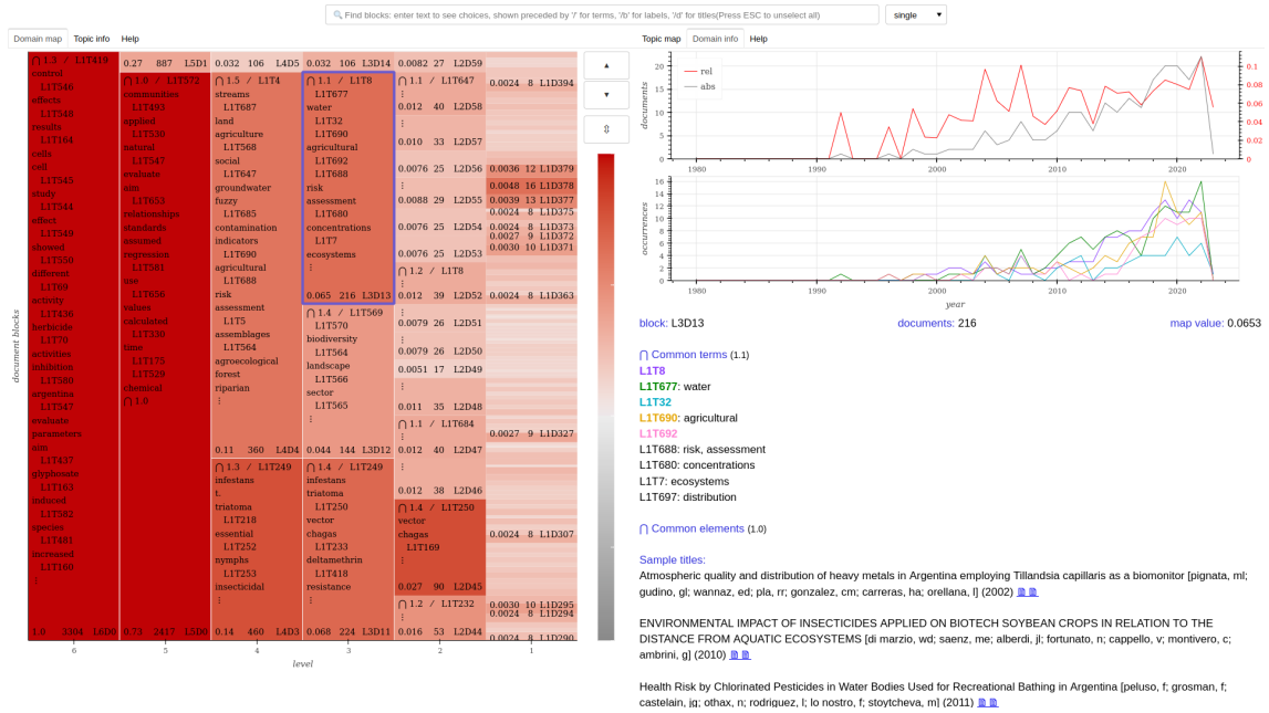
FIGURE 2 – Diagramme de blocs interactif. À gauche la partition multi-niveau d’un ensemble de documents inférée par un modèle à blocs stochastique. A droite l’évolution temporelle du bloc de niveau 3 sélectionné et des topiques qui le caractérisent, puis un échantillon de documents qu’il contient.
